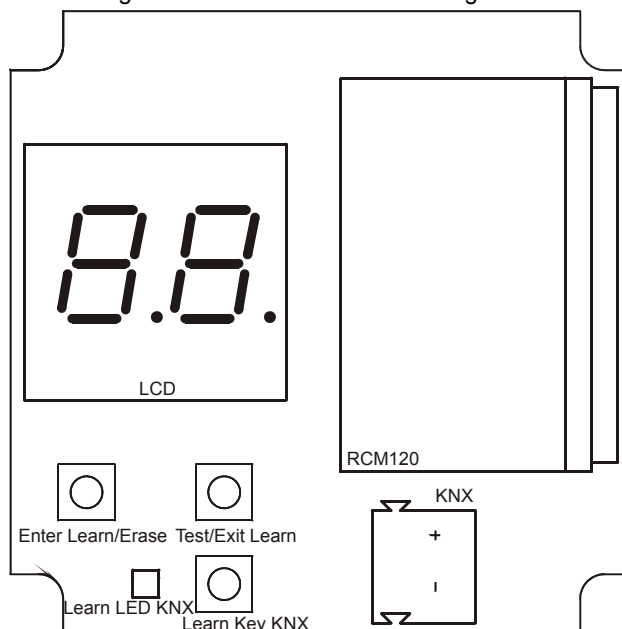
Abbildung 2: Oberseite des geöffneten Geräts
